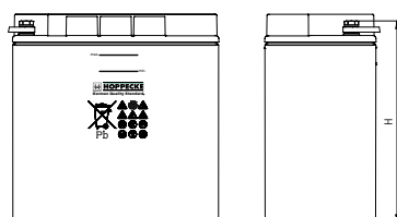
Fig. B Série OPzS bloc
